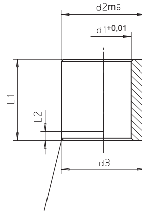
Zentrieransatz chamfer or centering neck
