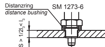
Form AK / AKN Form AKNN
