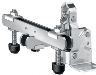
Montage über den Spannern / fitted above the clamping arm
