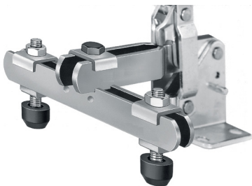
Montage unter den Spannern / fitted below the clamping arm
