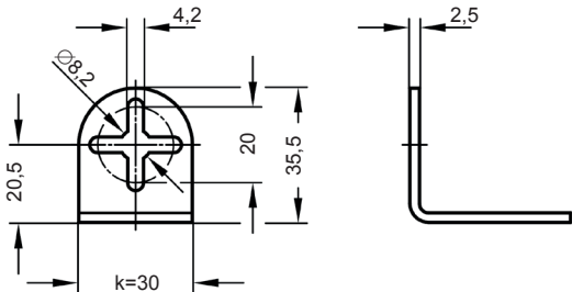
Laschenbreite k=30 / swivel width
