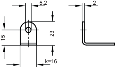
Laschenbreite k=16 / swivel width
