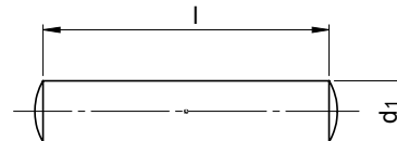
Zylinderstift DIN 7 dowel pin DIN 7
