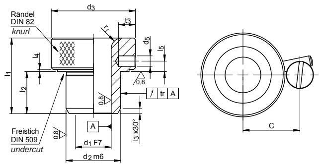
renewable drill bushes Steckbohrbuchse SM 1002-1 (als Schnellwechselbuchse)
