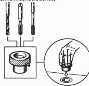
renewable drill bushes Steckbohrbuchse SM 1002-1 (als Schnellwechselbuchse)
