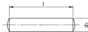
Zylinderstift DIN 7 dowel pin DIN 7
